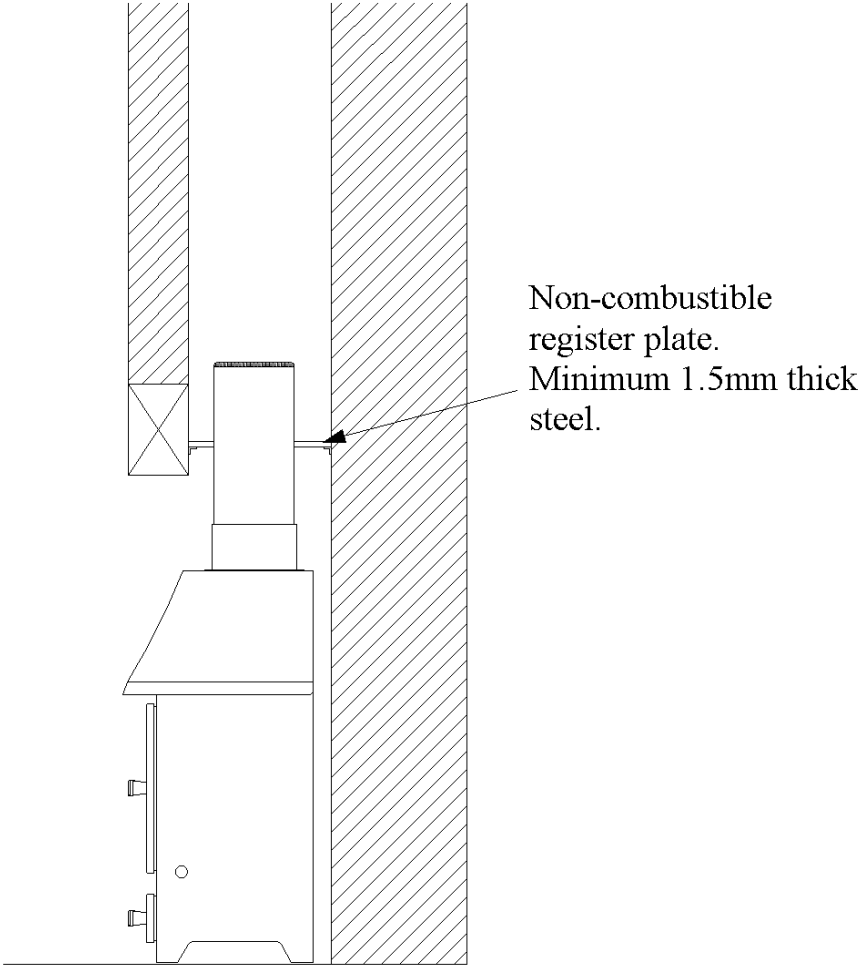
TOP FLUE OUTLET
